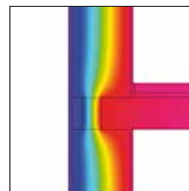
Visuelle Darstellung einer Wärmebrücke aus dem Wärmebrücken-Katalog von meinZiegelhaus
