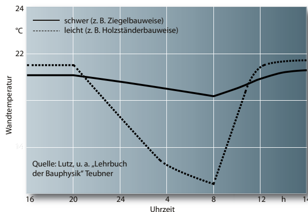
Auskühlverhalten eines Raumes
