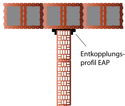
Schalloptimierte Anbindung einer leichten Trennwand
