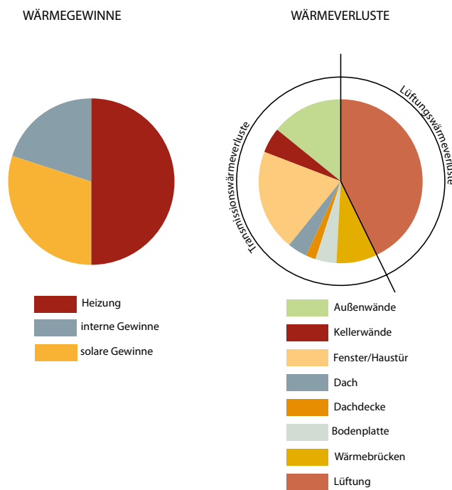
Verteilung von Wärmegewinnen und -verlusten für ein durchschnittliches Gebäude
