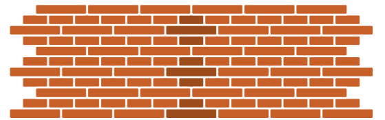
Kreuzverband
