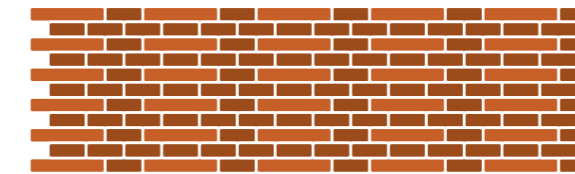
Holländischer Verband
