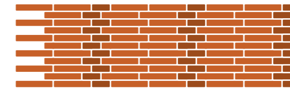
Schlesischer Verband
