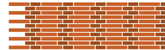
Gotischer Verband
